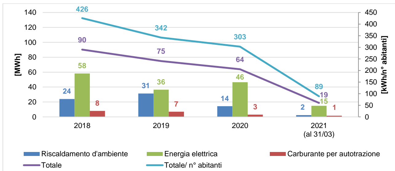
Grafico 1: Andamento dei consumi energetici del Comune nel periodo 2018 – 2021
