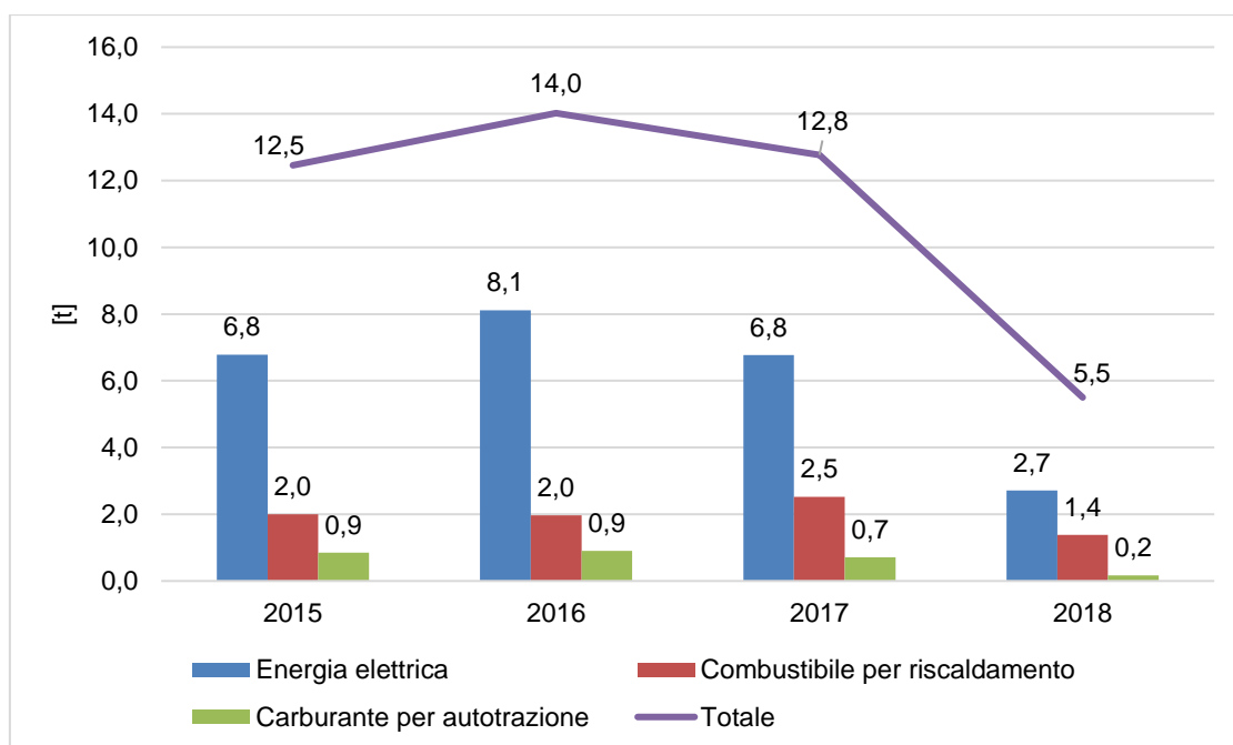
Grafico 2: Andamento delle emissioni di CO 2 nel periodo 2015-2018.
