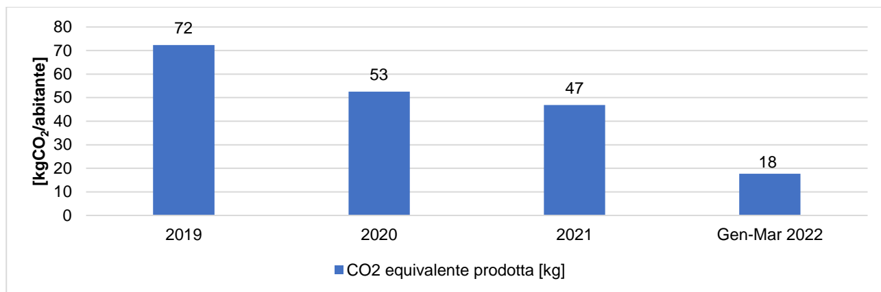
Grafico 2: Andamento delle emissioni di CO 2 nel periodo 2019-2022
