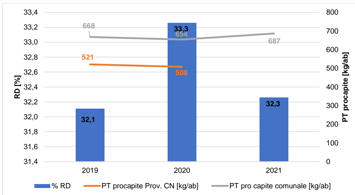
Grafico 4: Percentuale di raccolta differenziata e produzione totale pro capite di rifiuti nel periodo 2019 – 2021
