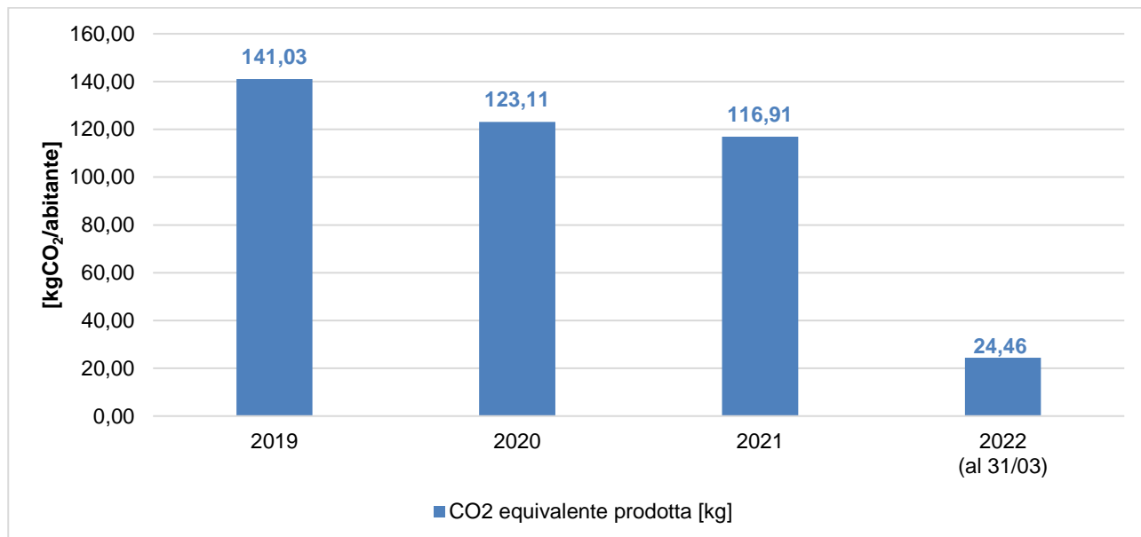
Grafico 2: Andamento delle emissioni di CO 2 nel periodo 2019-2022
